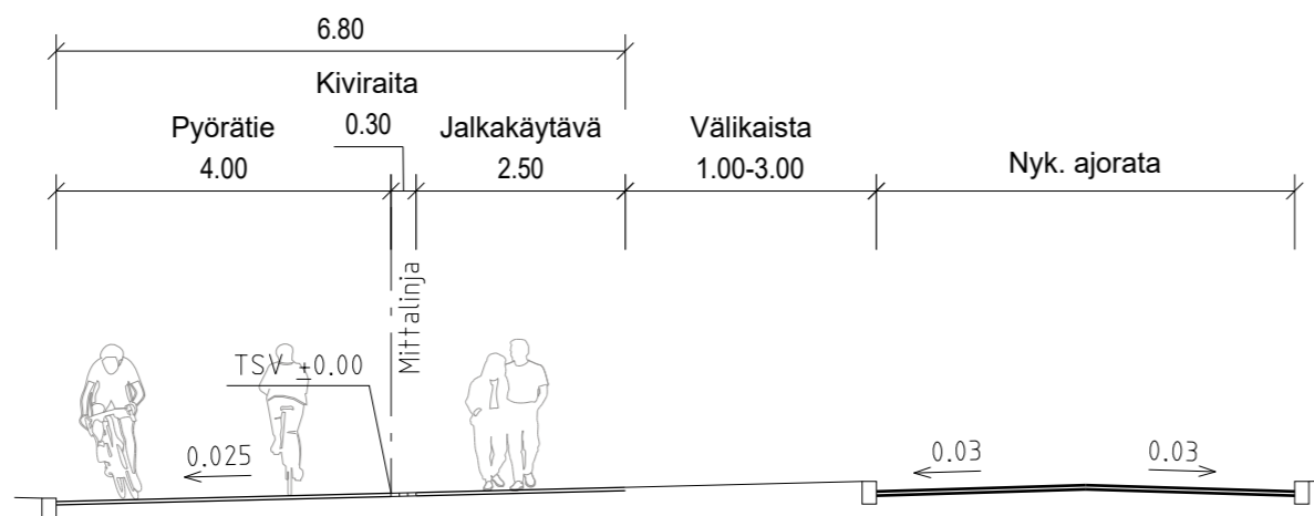
TYYPPIPOIKKILEIKKAUS, ESPOO RUOTUTORPPA PL 1140
