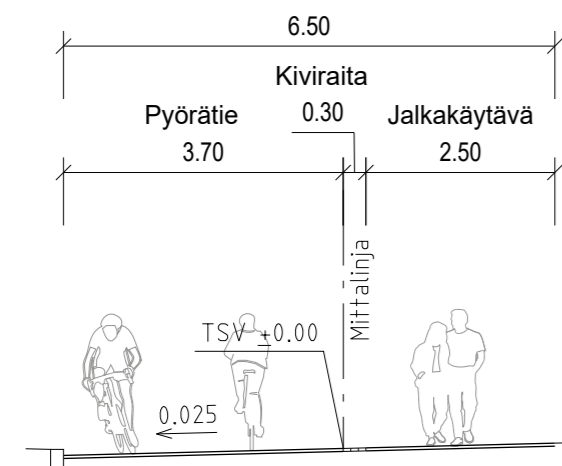
TYYPPIPOIKKILEIKKAUS, ESPOO KILON KALLIOLEIKKAUKSEN OSUUS (LR-ALUE), PL 520
