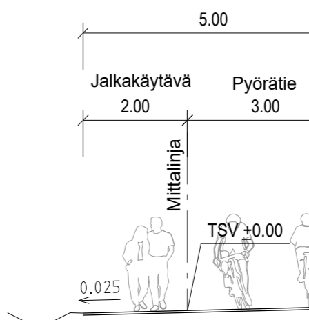
TYYPPIPOIKKILEIKKAUS, ESPOO VÄLI VADETINPORTTI-LASIIHTIN AK-ALUE (LR-ALUE) PL 10800
