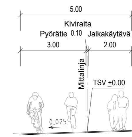
TYYPPIPOIKKILEIKKAUS, KAUNIAINEN PUISTO- JA EV-ALUE PL 4140
