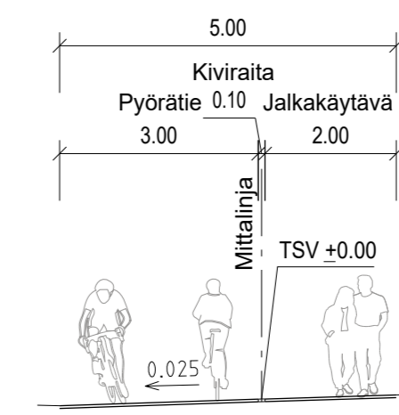
TYYPPIPOIKKILEIKKAUS, KAUNIAINEN LR-ALUE PL 6080
