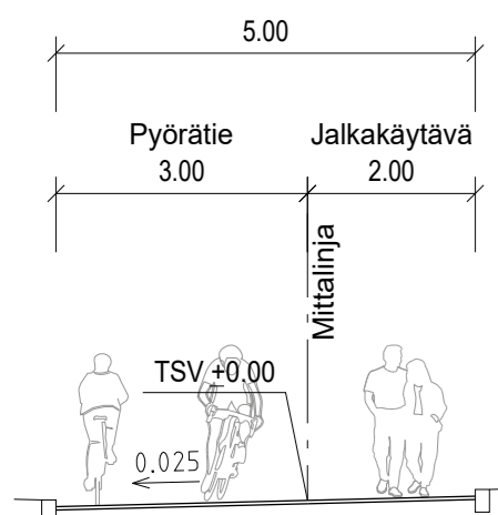
TYYPPIPOIKKILEIKKAUS, ESPOO TUOMARILA (LR-ALUE) PL 7070
