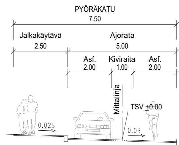
TYYPPIPOIKKILEIKKAUS, ESPOO HIIDENTIE PL 2340
