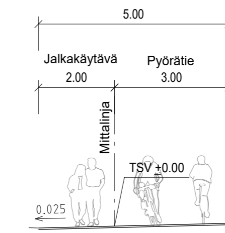
TYYPPIPOIKKILEIKKAUS, ESPOO MIKKELÄNPELTO PL 9600
