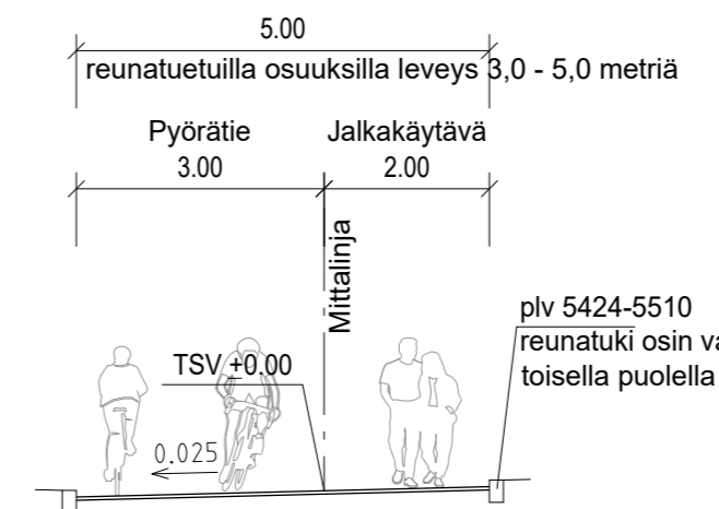
TYYPPIPOIKKILEIKKAUS, KAUNIAINEN REUNATUELLISET OSUDET PLV 3705-3895, 4235-4275, 5460-5510 JA 5995-6020
