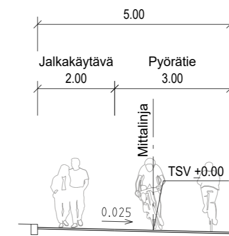
TYYPPIPOIKKILEIKKAUS, ESPOO JOKITÖRMÄ PL 9100
