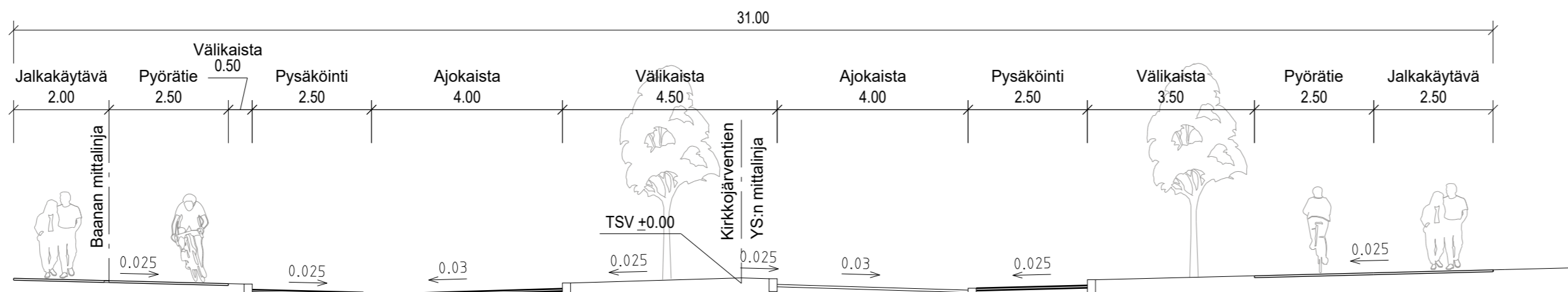
TYYPPIPOIKKILEIKKAUS, ESPOO KIRKKOJÄRVENTIE
